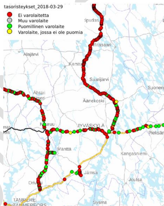
Kuva 6 Keski-Suomen rataverkko ja tasoristeykset (Lähde Väylä.fi)
