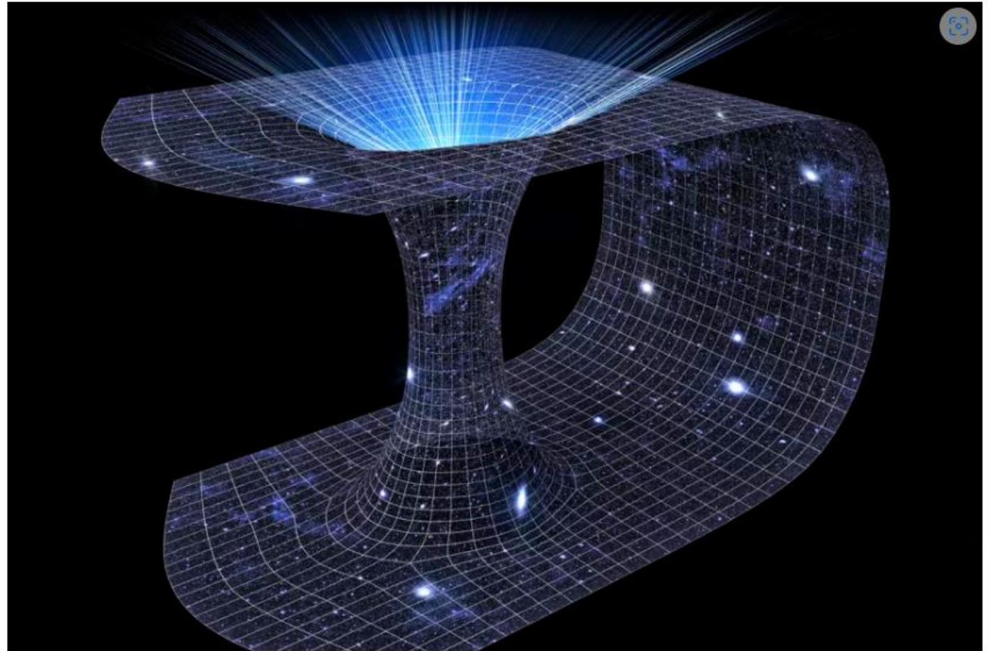
Taiteilijan kuvitelma madonreistä, joka muodostaa oikotien neliulotteisen aika-avaruuden kahden pisteen välillä.
